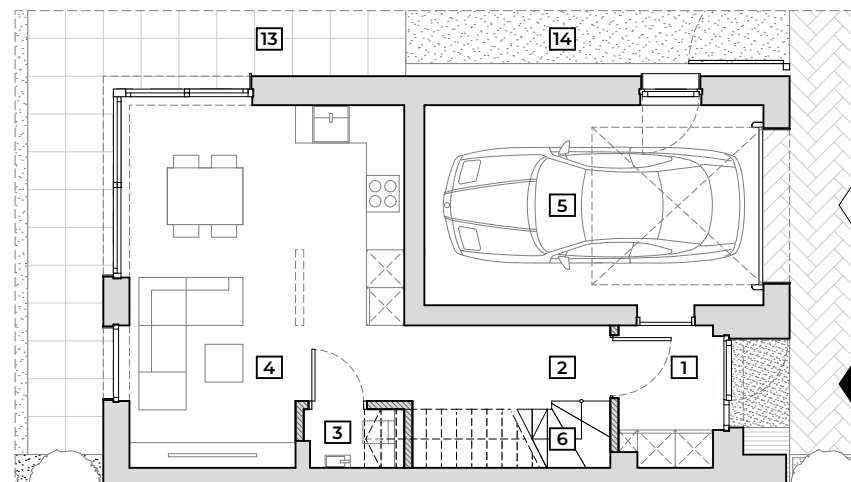
RZUT PARTERU
