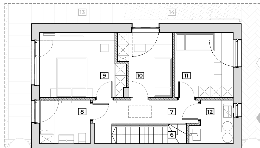
RZUT PIĘTRA
